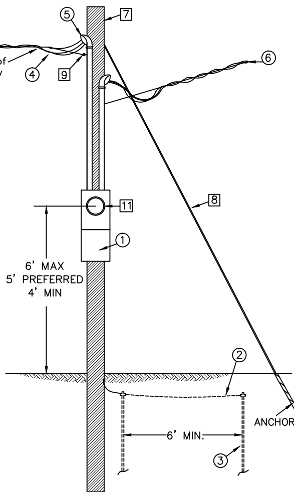
OVERHEAD-OVERHEAD
